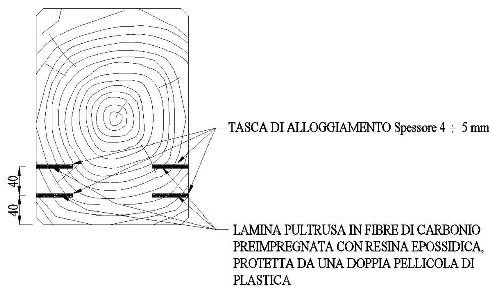
Figura 105. Rinforzo di elemento in legno mediante lamine pultruse inserite in tasche laterali su doppio registro
