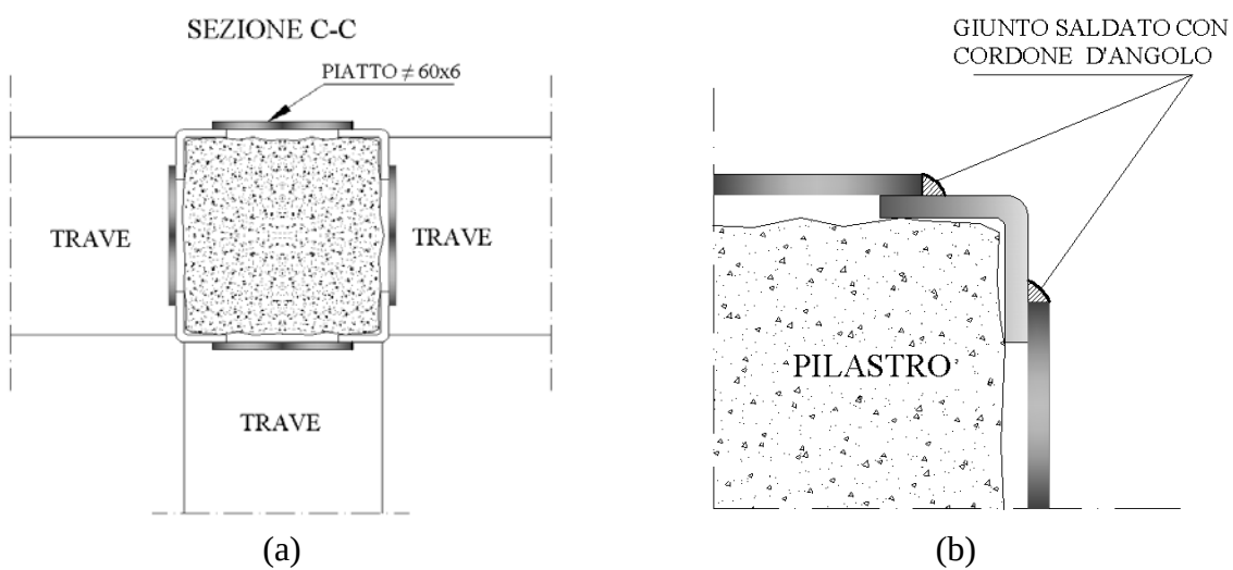
Figura 40. Viste in sezione: (a) sezione C-C (b) particolare della saldatura con cordone d'angolo
