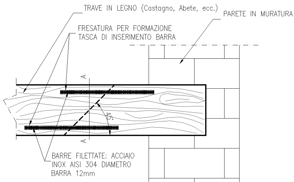
(a) SEZIONE A-A
