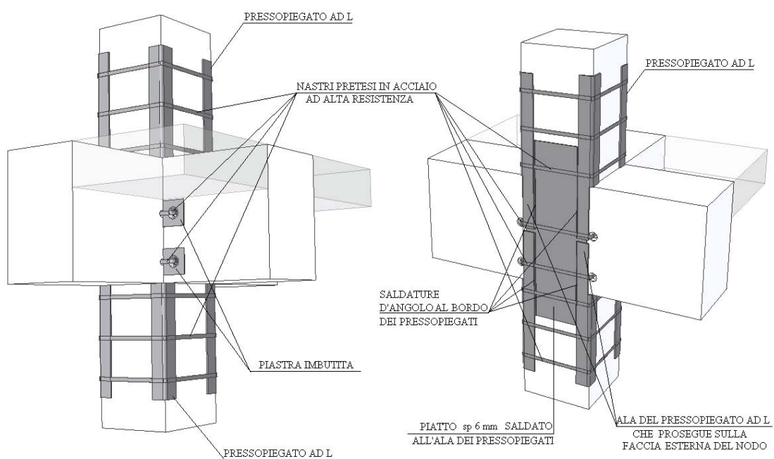
Figura 31. Pressopiegati ad L, piastra e nastri pretesi in un nodo intermedio
