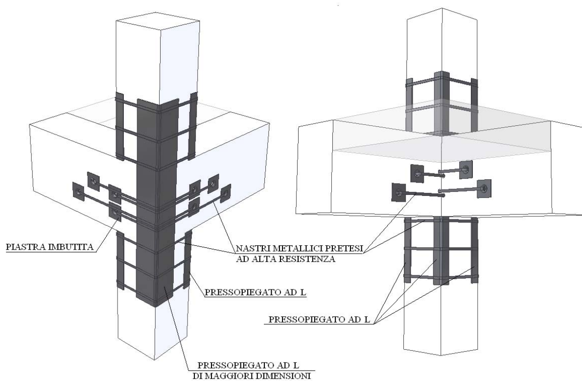
Figura 29. Pressopiegati ad L e nastri pretesi in un nodo d'angolo
