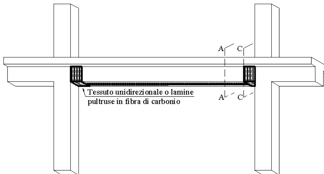
Figura 81. Rinforzo a flessione con compositi di una trave in c.a. con ancoraggi di estremità
